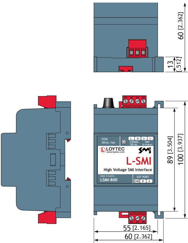
DIM033 LSMI-800
