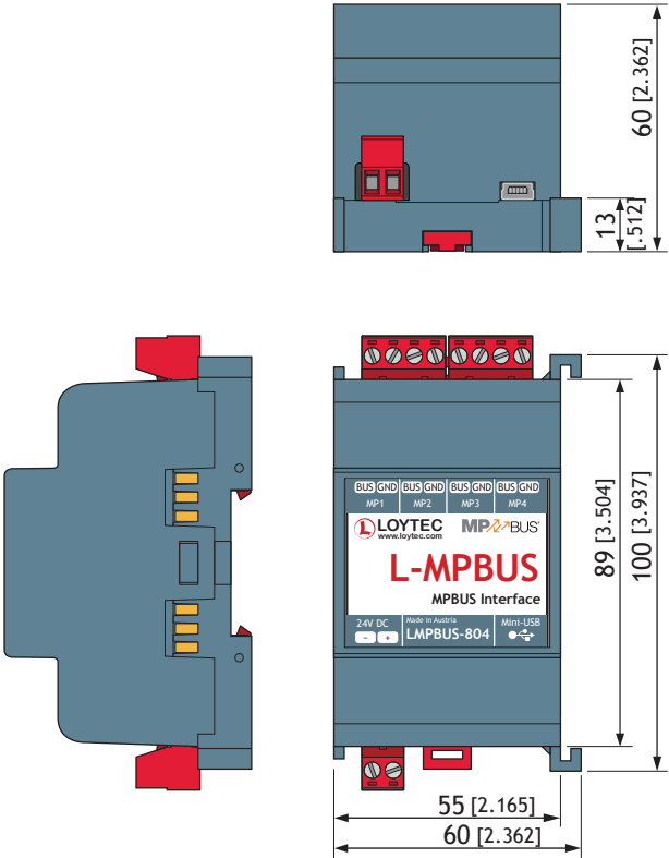
DIM051 LMPBUS-804
