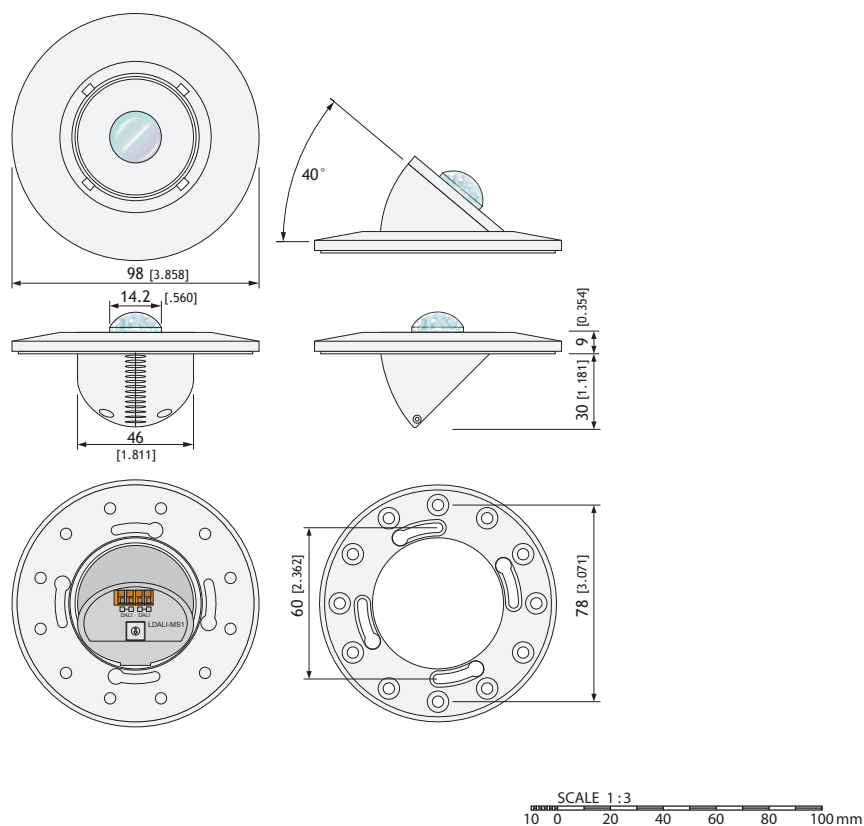
DIM042 LDALI-RM1 LDALI-RM2
