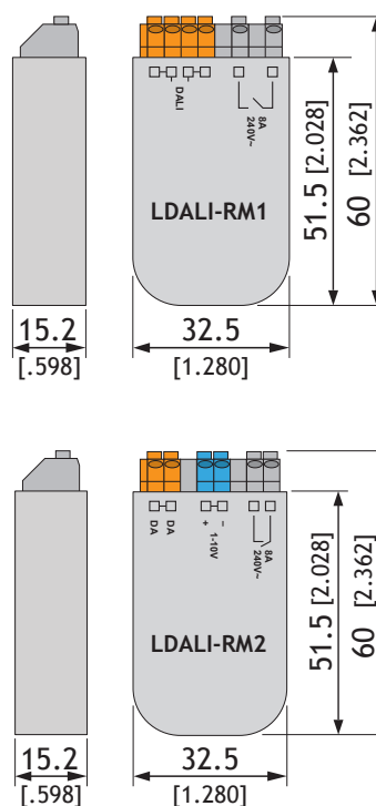
DIM042 LDALI-RM1 LDALI-RM2
